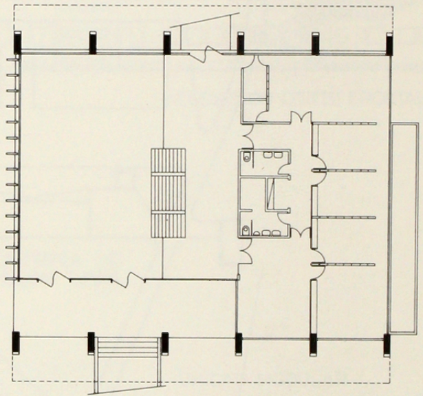
PLANTA BLOQUE A 1° P
