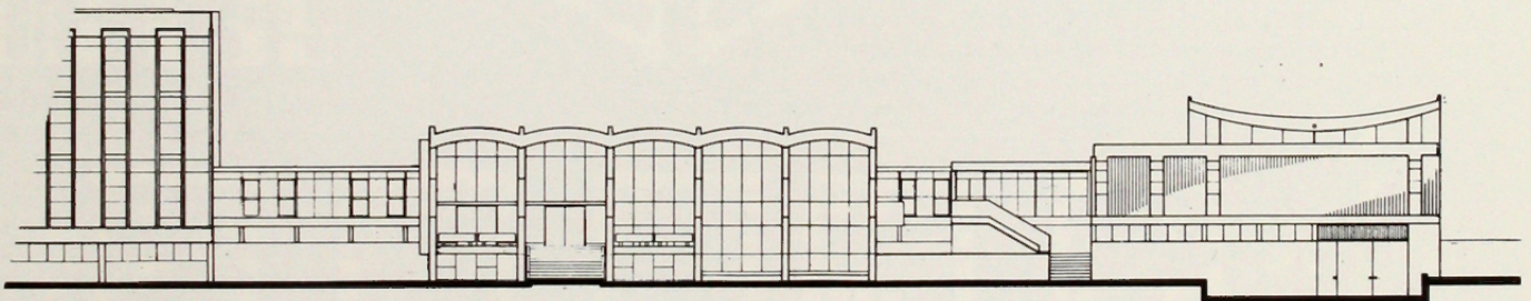
ELEVACION SUR BLOQUES A Y C
