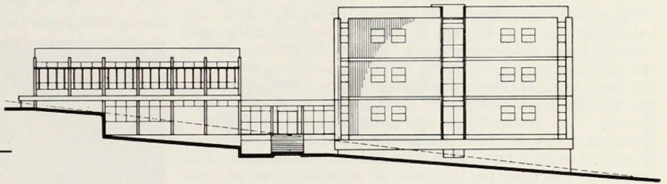
ELEVACION PONIENTE BLOQUE B Y D
